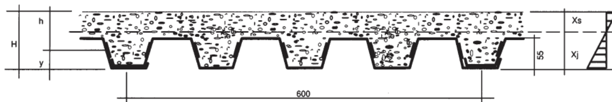
CARATTERISTICHE STATICHE DELLA SOLETTA m = 10
