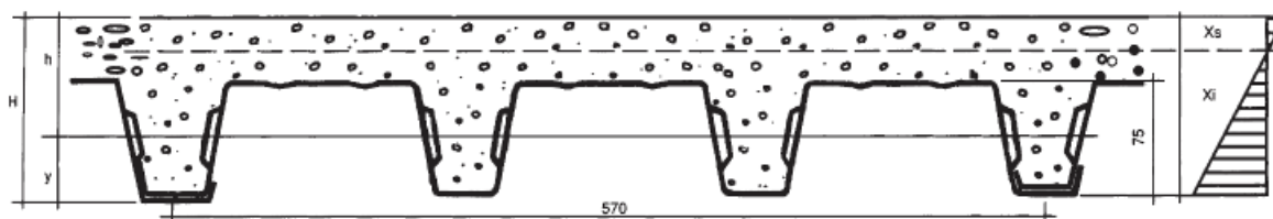
CARATTERISTICHE STATICHE DELLA SOLETTA m = 10
